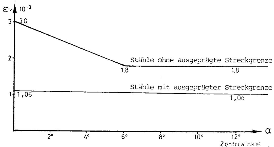
Darstellung 1: Zulässige Vergleichsdehnungen \epsilon_v im meistbeanspruchten Leitungsquerschnitt in Abhängigkeit vom Zentriwinkel \alpha
