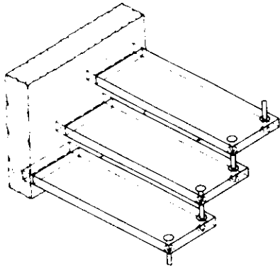
Bild 1. Einbolzentreppe WE 1
