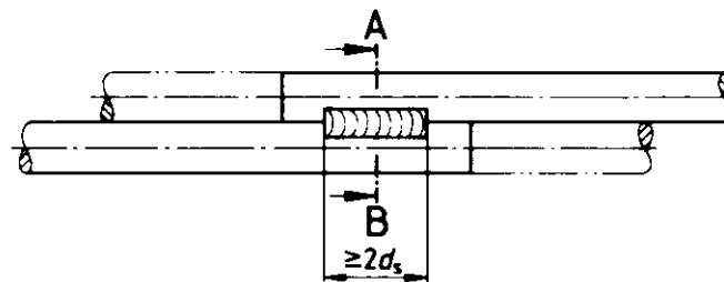
Bild 2. Überlappstoß als nichttragende Verbindung ( d_s Nenndurchmesser des gegebenenfalls dünneren der gestoßenen Stäbe)
