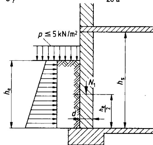
Bild 3. Lastannahmen für Kellerwände
