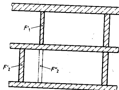
Bild 3. Versetzt angeordnete flankierende Wände F_1 und F_2 Ausnahmefall, für die Berechnung der Korrekturwerte wird anstelle der Wand F_2 die Wand F''_2 angenommen
