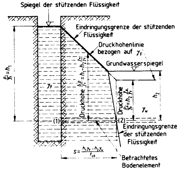
Bild 10. Auf die Wichte der stützenden Flüssigkeit \gamma_F bezogenes Druckhöhengefälle im betrachteten Bodenelement
