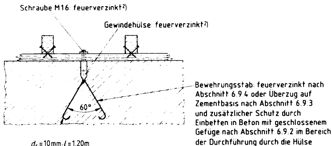
Bild 2. Deckenanschluß
