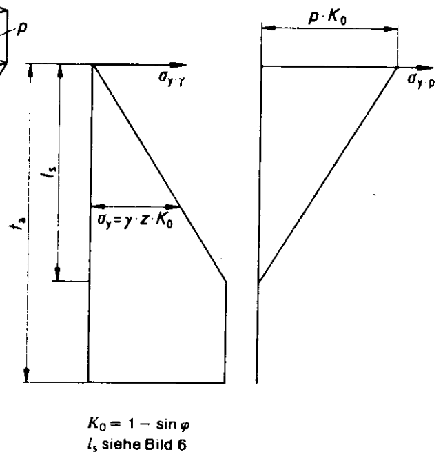
Bild 7. Näherung für den Bruchkörper, Ansatz der stützenden Schubspannungen in den dreieckförmigen Flankenflächen des Bruchkörpers
