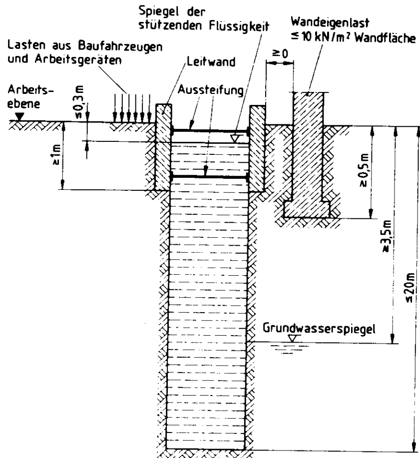
Bild 9. Schlitz mit einer Länge l_s \leq 3,5 m mit unmittelbar an den Schlitz angrenzenden Gebäuden
