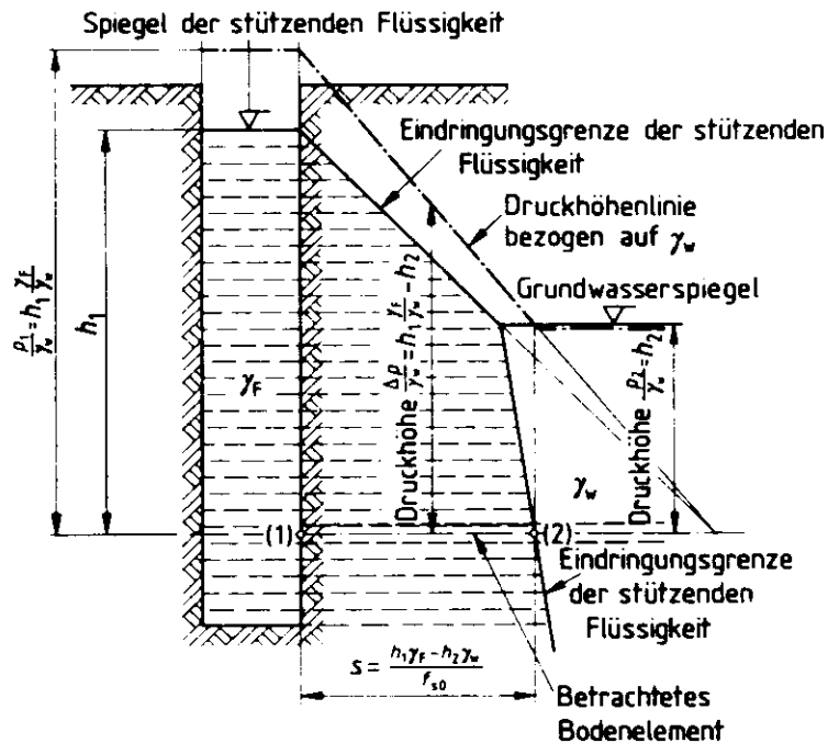
Bild 11. Auf die Wichte des Wassers \gamma_w bezogenes Druckhöhengefälle im betrachteten Bodenelement
