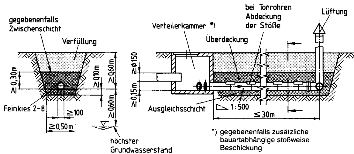
Bild 5. Untergrundverrieselung, Schnitte
