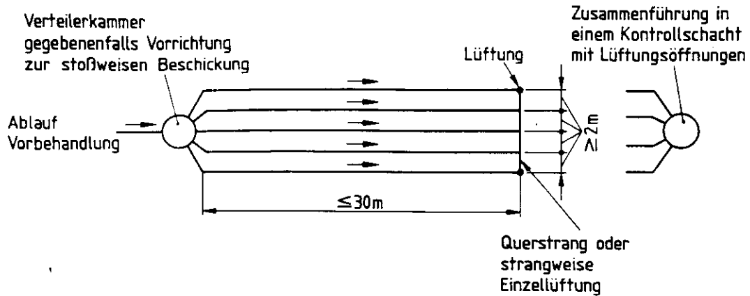
Bild 4. Anordnung einer Untergrundverrieselung
