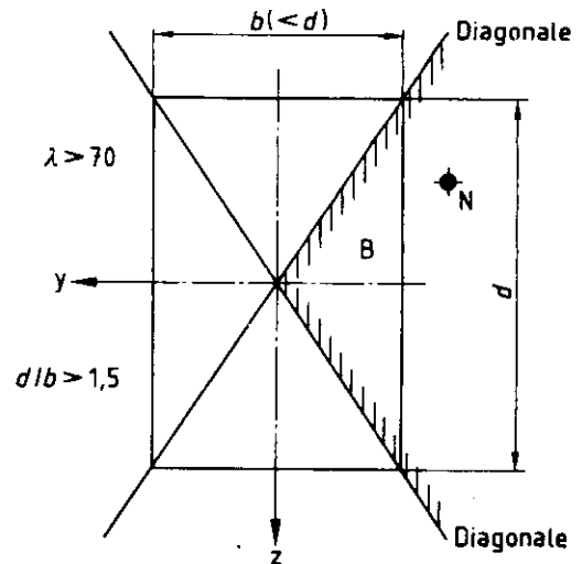
Bild 14.1. Rechteckquerschnitt unter schiefer Biegung mit Längsdruck; Anwendungsgrenzen für das Näherungsverfahren nach Abschnitt 17.4.8 b) für d/b > 1,5 und \lambda > 70
