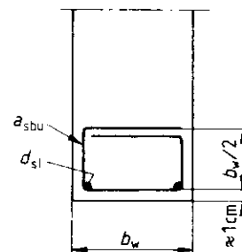
Bild 43. Zusätzliche Querbewehrung
