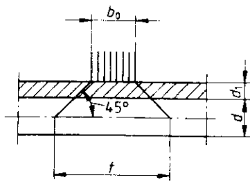
Bild 44. Lasteintragungsbreite
