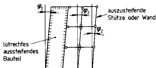
Bild 9. Schiefstellung \varphi_2 aller auszusteifenden und aussteifenden lotrechten Bauteile
