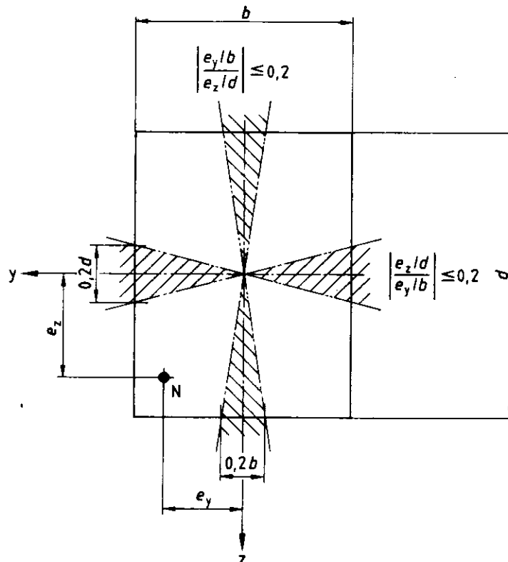
Bild 14.2. Rechteckquerschnitt unter schiefer Biegung mit Längsdruck; Anwendungsgrenzen für das Näherungsverfahren
