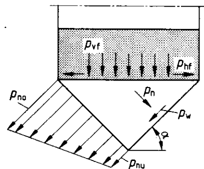
Bild 4. Lasten aus der Trichterfüllung
