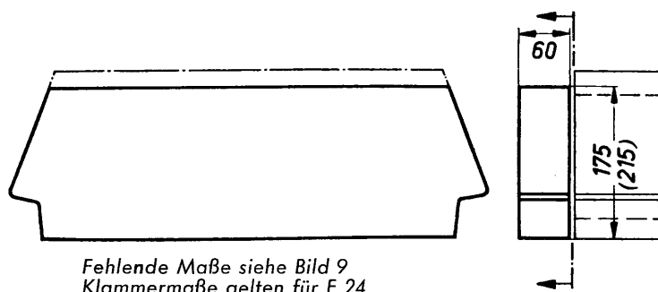
Bild 10 Abmessungen der Abschlußsteine
