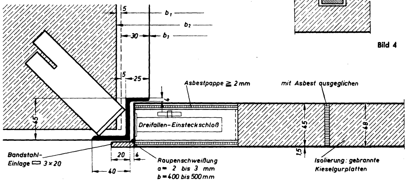
Schnitt A-B
