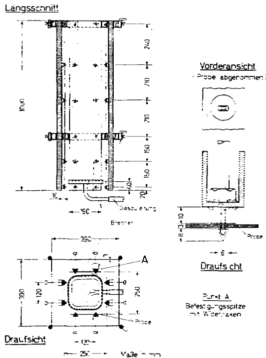
Abb. 1 Aufbau der Prüfkörper aus flexiblem Material Befestigung der Proben an der Haltevorrichtung und Anordnung des Ringbrenners. Maße in mm.
