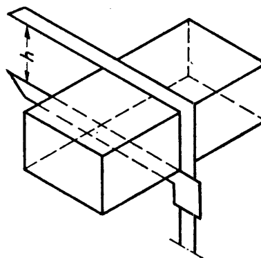
Bild 17. Höhenmessung 2
