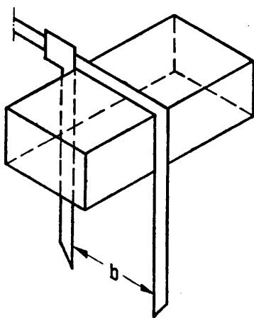
Bild 12. Breitenmessung 1
