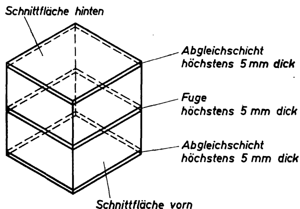
Bild 20. Probewürfel aus gehälfteten Vollziegeln
