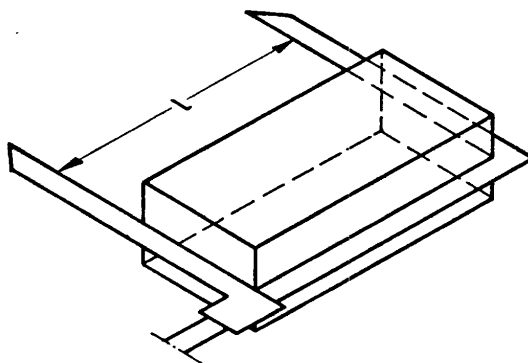
Bild 15. Längenmessung 2
