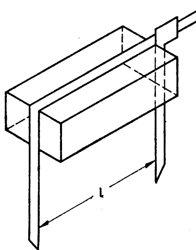
Bild 14. Längenmessung 1
