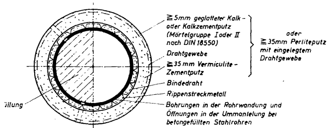
Bild 4: Stahlrohrstütze mit Ummantelung aus Vermiculite-Zementputz oder Perlite-Zement- bzw. Gipsputz auf Rippenstreckmetall
