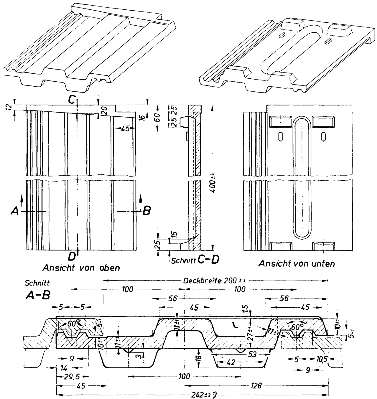
Bezeichnung: Falzdachstein B DIN 1117
