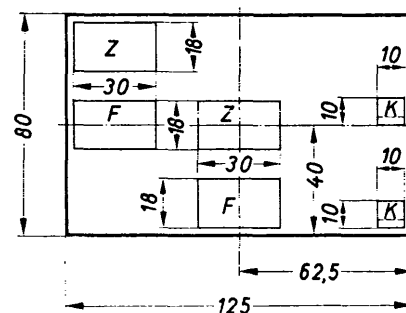
Bild 10. Prüfstück Nr 13
