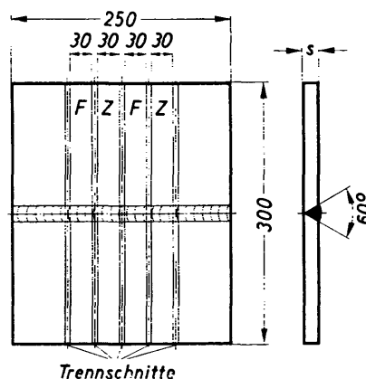
Bild 7. Prüfstück Nr 11
