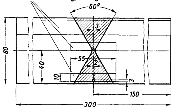
Bild 9. Prüfstück Nr 13
