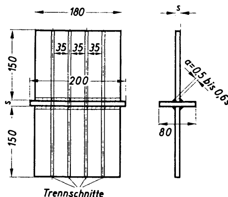
Bild 8. Prüfstück Nr 12
