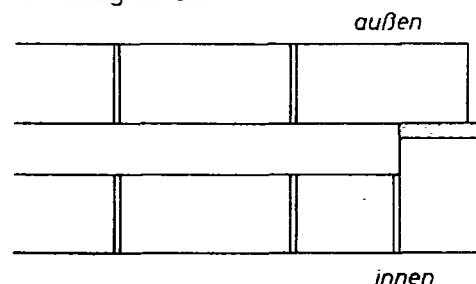
Bild 5. Sperrschicht in Fensteranschlüssen
