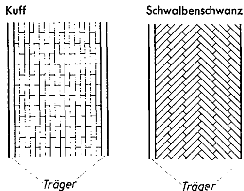
Bild 6. Gewölbeverbände
