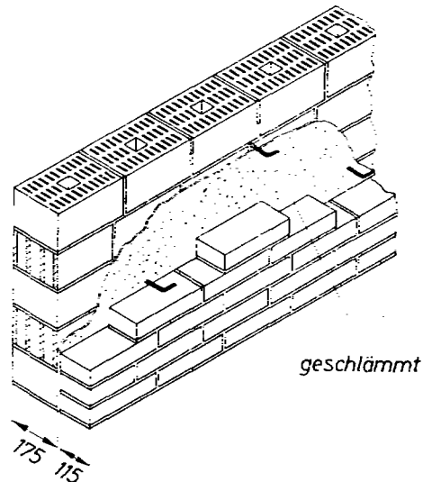
Bild 7. Verblendmauerwerk mit Hintermauerung in größerformatigen Lochsteinen.
