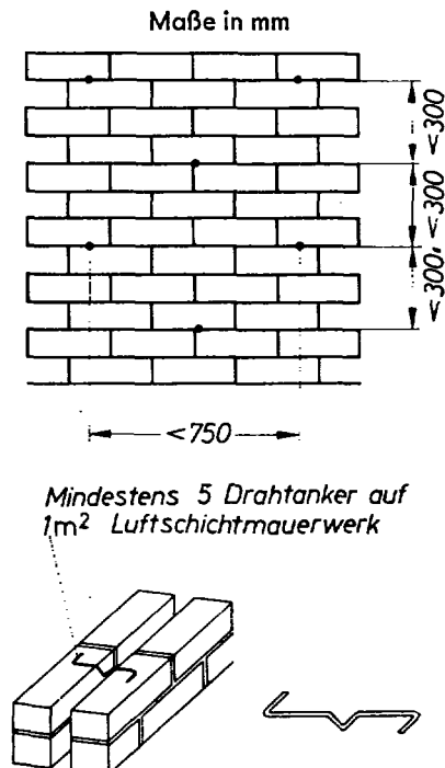
Bild 3. Drahtanker für Hohlmauerwerk
