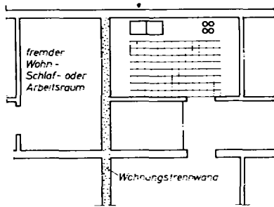
Armatur oder Rohrleitung in der Nähe der Wohnungstrennwand, deshalb Grundriss - Anordnung I
