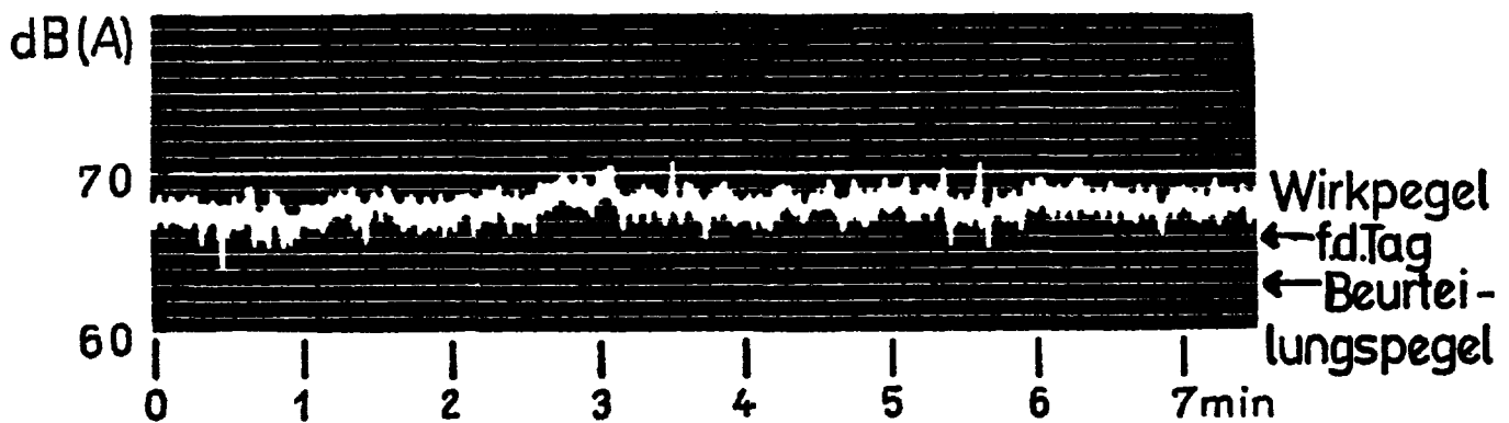
Bild 9: Ermittlung eines Beurteilungspegels für einen einschichtig arbeitenden Betrieb
