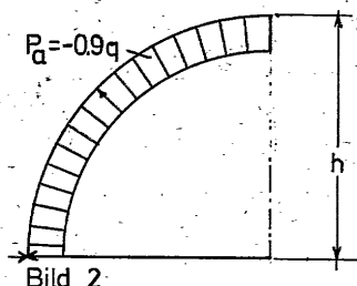
Bild 2 Vereinfacht angenommene Belastung einer Viertelkugel durch Windsog
