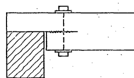
Bild 14. Sicherung eines Balkenaufagers gegen Aufreißen
