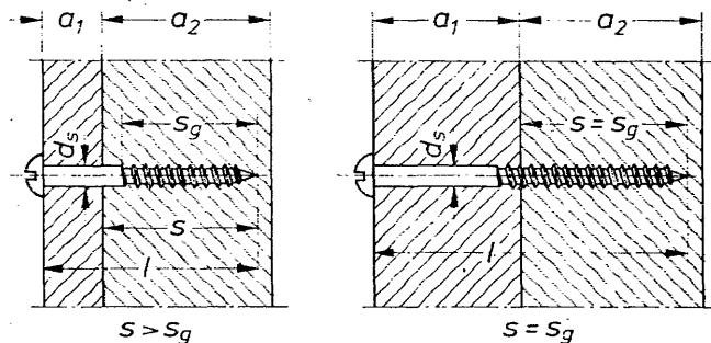
Bild 25. Holzdicke und Einschraubtiefe bei Holzschrauben
