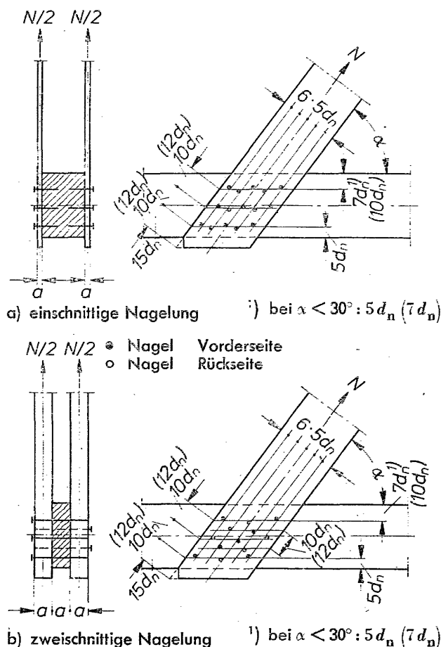
Bild 22. Mindestnagelabstände nicht vorgebohrter Nagelungen
