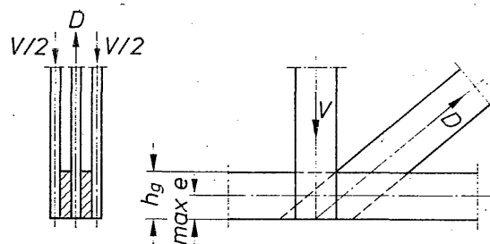
Bild 2. Ausmittiger Stabanschluß mit e = h_g/2
