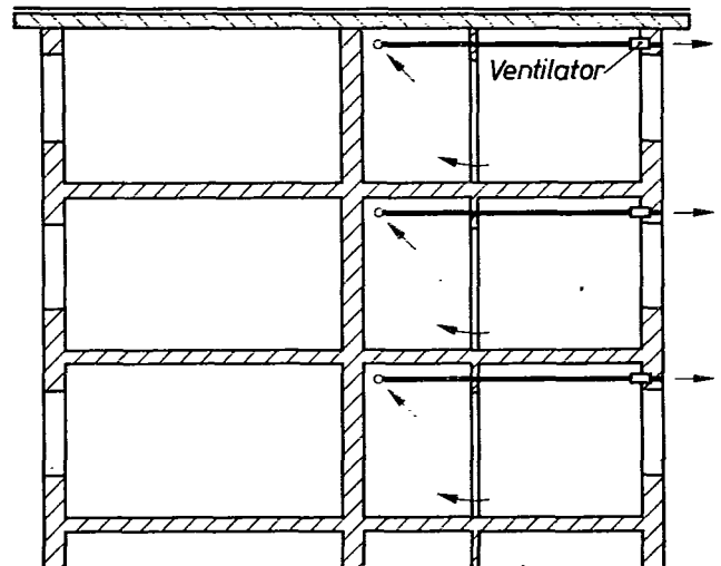
Bild 2. Einzelentlüftungsanlagen mit seitlicher Abfuhr der Abluft
