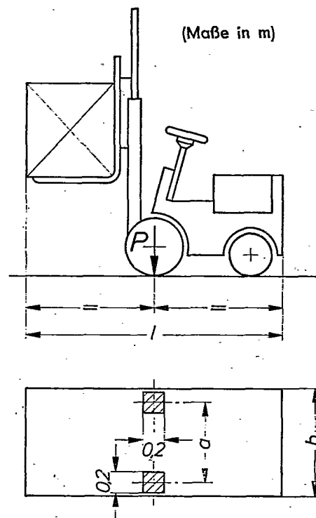
Bild 1. Abmessungen der Gabelstapler
