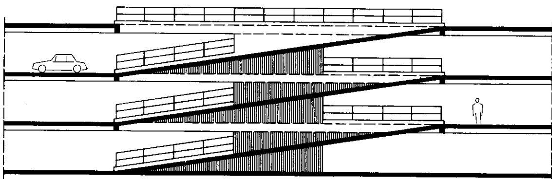
BILD 3 Seitliche Trennwände zwischen Geschoßdecken und Rampenoberseiten und -unterseiten
