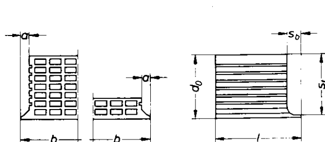
Bild 5. Deckenziegel für den Bereich negativer Momente
