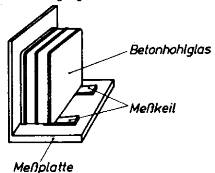
Bild 1. Meßanordnung für Prüfung bei Betonhohlgläsern
