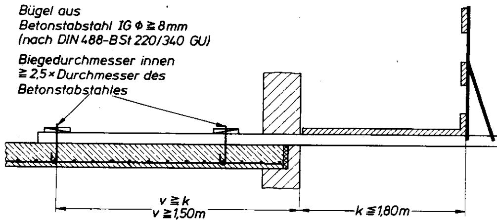
Bild 11. Auslegerbefestigung
