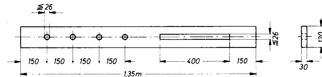
Leiterholmverlängerung (LHV)
