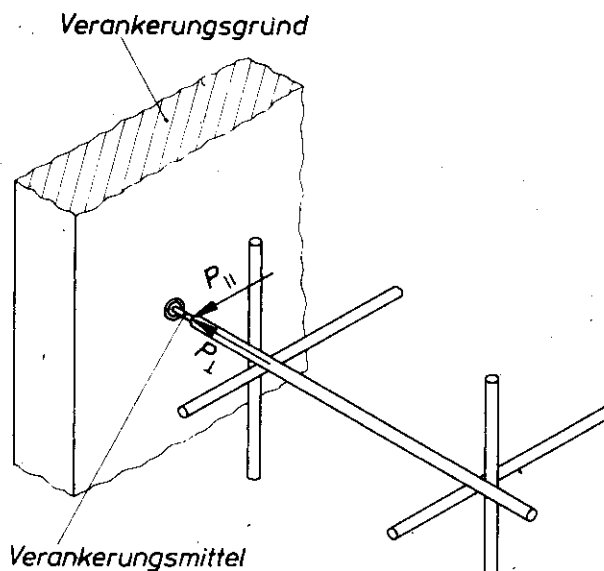
Bild 3. Darstellung der Ankerkräfte (Die dargestellten Kräfte können sowohl in positiver als auch in negativer Richtung auftreten).
