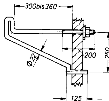
Konsole für eine Bohle (verschraubt) (K1S1)
