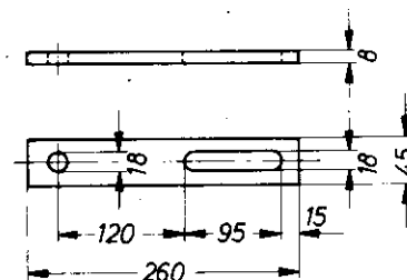
Querlasche (QLS)
