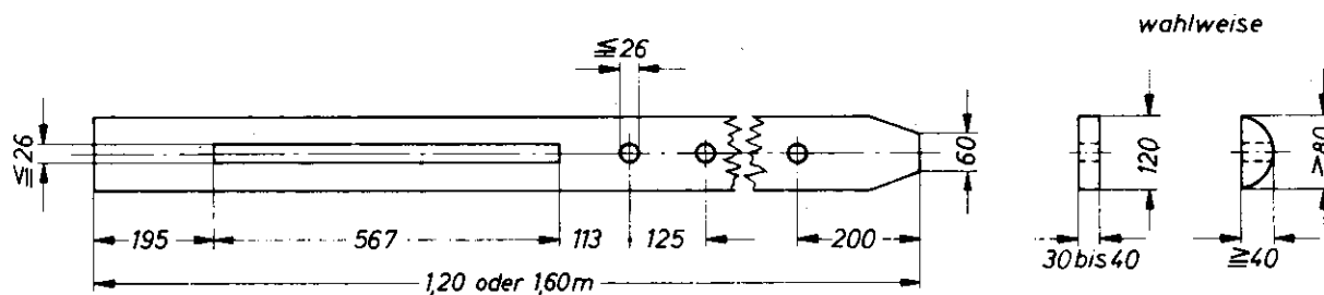
Dübelarm (DAF und DAR)
