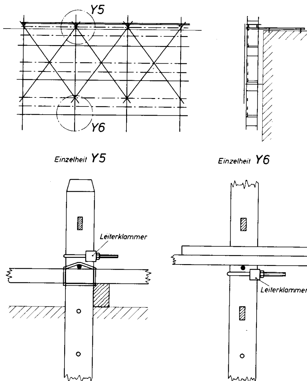
Bild 8. Hängendes Leitergerüst
