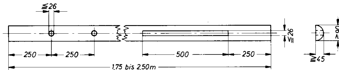
Leiterholmverlängerung (LHV)
