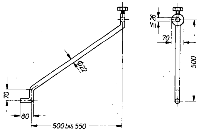
Konsolstrebe für zwei Bohlen (KST 2)
