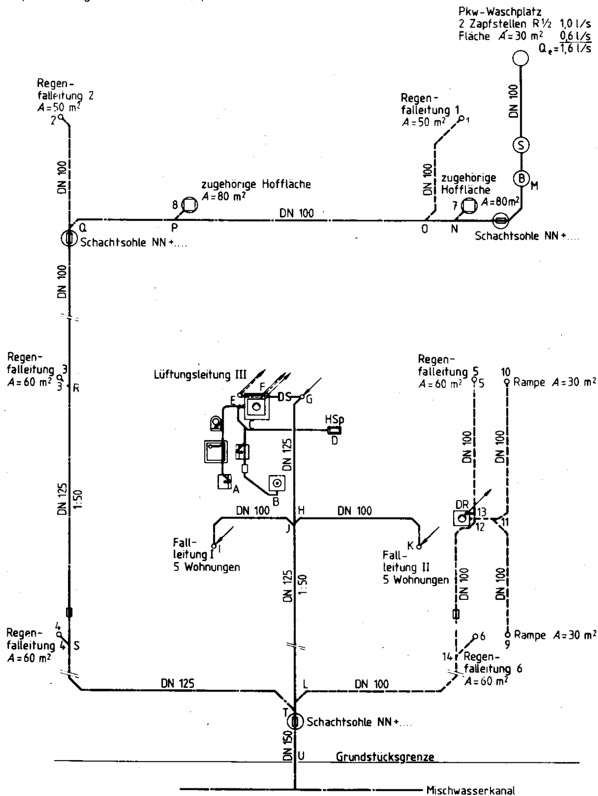
Bild A.3 Mischverfahren
