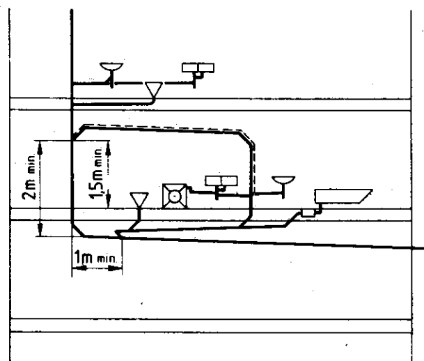
Bild 10. Umlüftung von Sammelanschlussleitung auf Fallleitung
