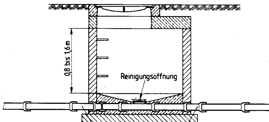
Beispiel für gelenkigen Anschluß
