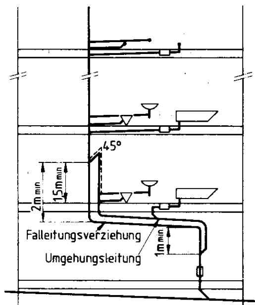
Bild 7. Falleitungsverziehung mit Umgehungsleitung
