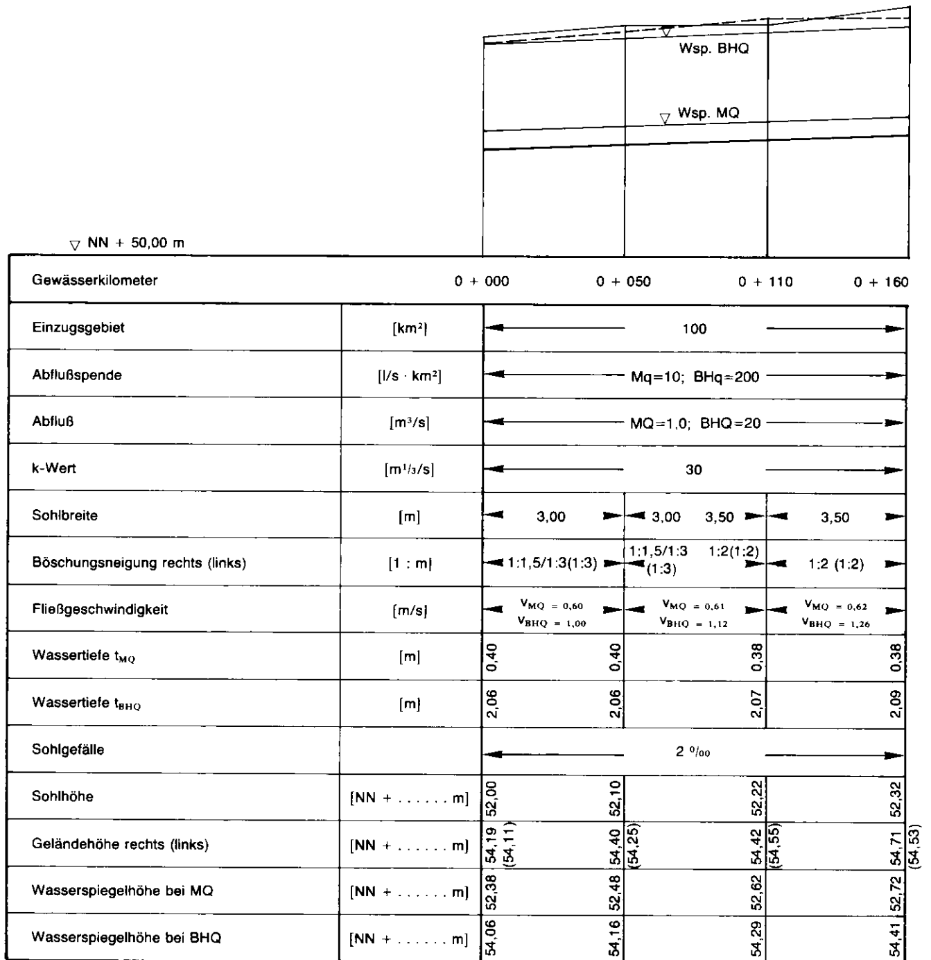
Abb. 10 Längsschnitt zum Berechnungsbeispiel
