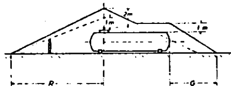
◀ Bild 4a: Beispiel einer Schutzzone für einen oberirdisch aufgestellten Behälter mit Einschränkung der Schutzzone durch eine Wand
