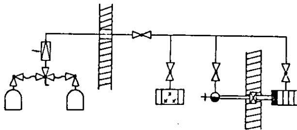
Bild 1: Flaschenanlage mit Entnahme aus der gasförmigen Phase
