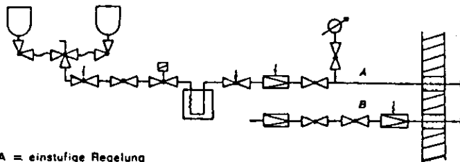
Bild 2: Flaschenanlage mit Verdampfer und Entnahme aus der flüssigen Phase
