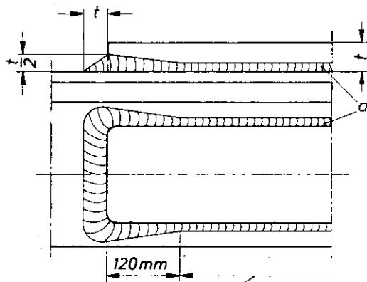
Bereich der Nahtdicke a nach Berechnung für Lamellenanschlüsse
