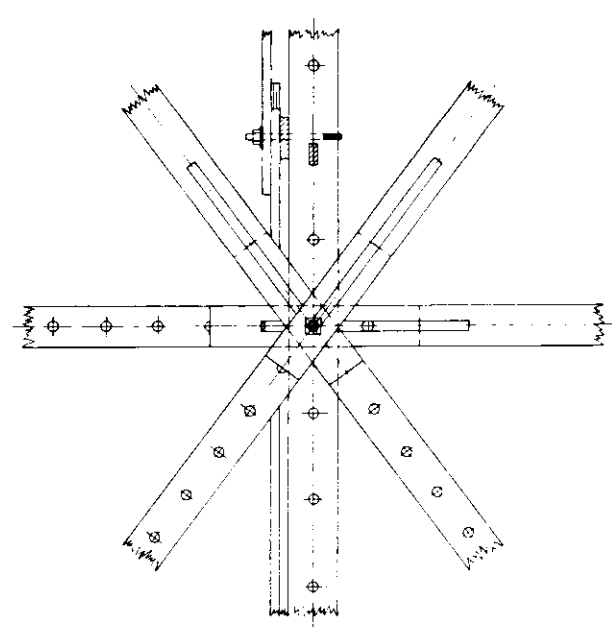
Einzelheit X3
