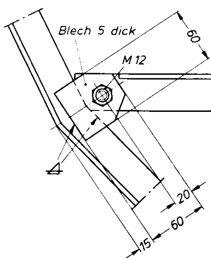
Einzelheit Y1
