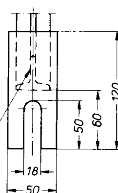
Einzelheit Y3
