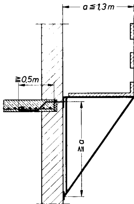
Lage der Bügel bei Doppelbefestigung
