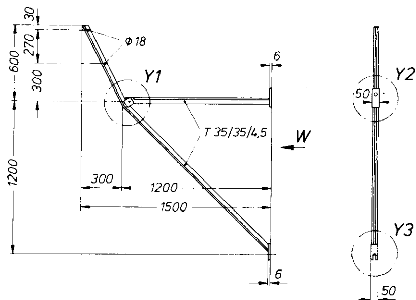
Ansicht W
