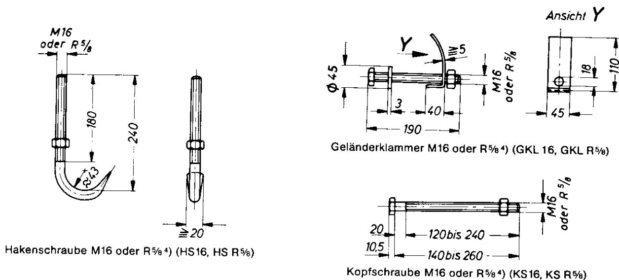
Bild 15. (Fortsetzung) Formen, Maße, Werkstoffe und Ausführungen von Gerüstbauteilen aus Holz nach Abschnitt 4.2.2 (Maße in mm)
