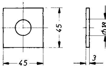
Unterlagscheibe für Kopf- und Hakenschrauben (USCH)
