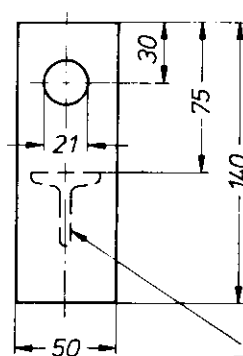
Einzelheit Y2
