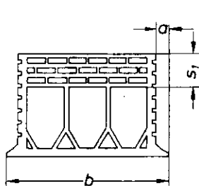
a) Querschnitt
