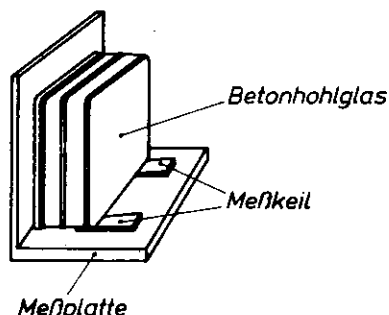
Bild. Meßanordnung für Prüfung bei Betonhohlgläsern
