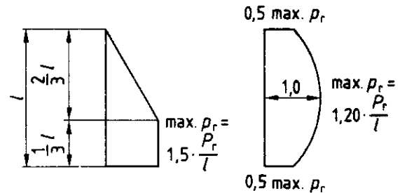
Bild 32. Verteilung der Ringzugkraft über die Länge des Verankerungskopfes
