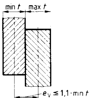
Bild 21. Überlappte Kreiszylinderschalen
