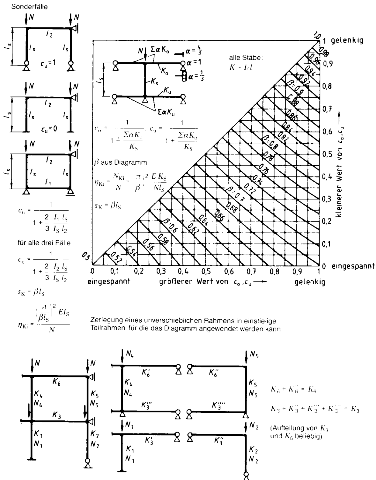
Bild 27. Diagramm zur Bestimmung des Verzweigungslastfaktors \eta_{Ki} und der Knicklängen s_K für Stiele unverschieblicher Rahmen mit \epsilon_{Riegel} \leq 0,3
