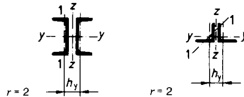
Bild 19. Mehrteilige Stäbe, deren Querschnitte eine Stoffachse haben und bei denen der lichte Abstand der Einzelstäbe nicht oder nur wenig größer ist als die Dicke des Knotenbleches
