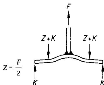
Bild 21. T-Stoß
