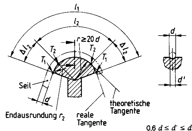
Bild 11. Endausrundung von Umlenkclagern
