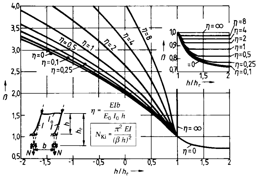
Bild 36. Knicklängenbeiwerte für den an den Stelfüßen gelenkig gelagerten Portalrahmen
