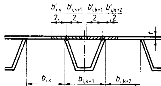
Bild 7. Wirksame Gurtbreiten von gedrückten Längssteifen
