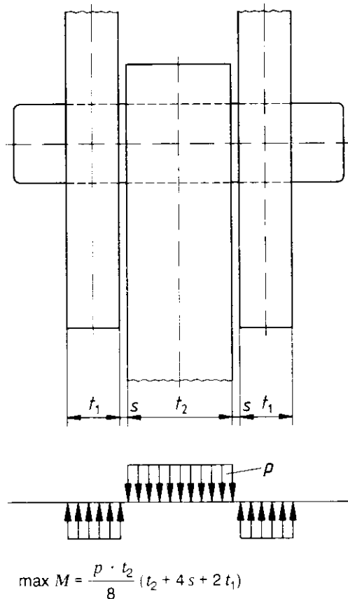
Bild 27. Ermittlung des Biegemomentes in einem Bolzen
