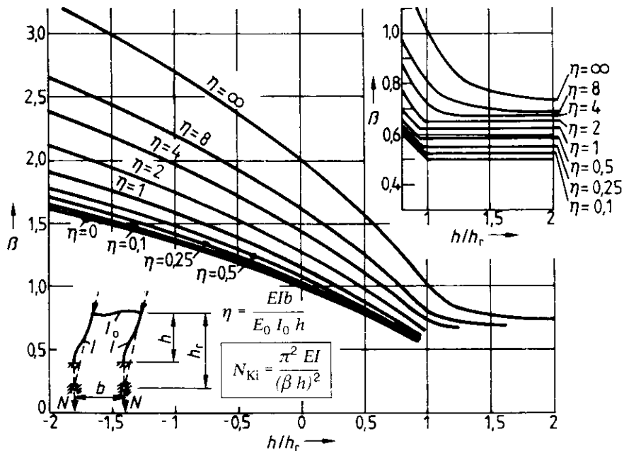
Bild 37. Knicklängenbeiwerte für den an den Stelfüßen einge- spannten Portalrahmen
