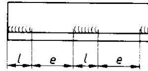
Bild 30. Zur Berechnung von Schweißnahtschubspannungen \tau_I in unterbrochenen Längsnähten
