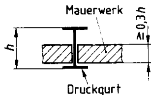
Bild 11. Aussteifung durch Mauerwerk
