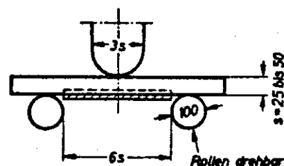
Bild 15. Aufschweißbiegeversuch
