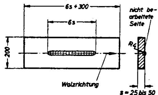
Bild 14. Probe für den Aufschweißbiegeversuch
