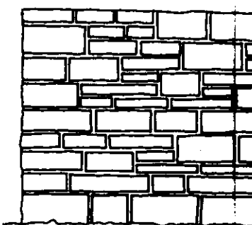
Bild 18. Unregelmäßiges Schichtenmauerwerk
